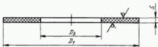
Размеры, мм
